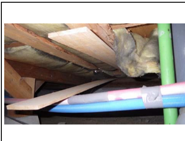
撮影箇所:22 床断熱押え部材欠落
